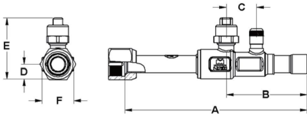
图纸 B
